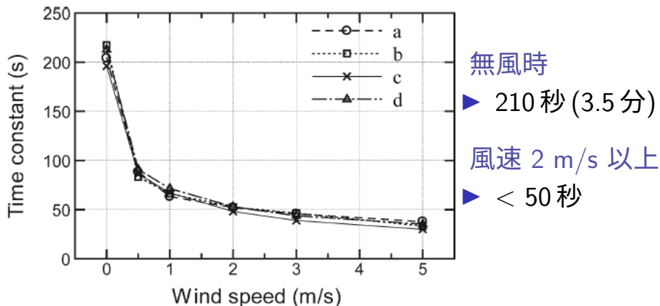
第 4 図 温度計の時定数と通風速度との関係。
